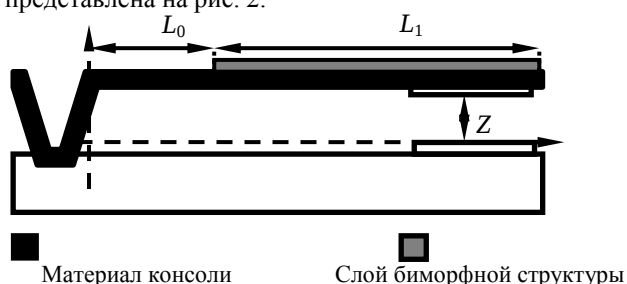
Рис. 2. Схема термочувствительного элемента
