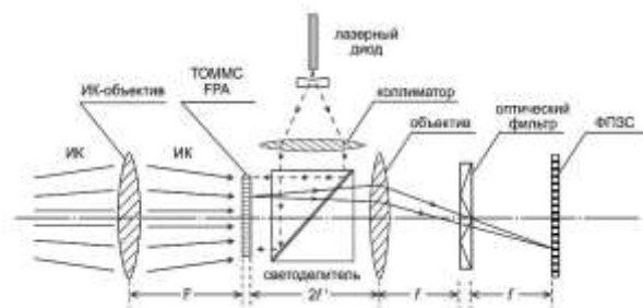
Рис. 1. Схема ИК ТМСОС
