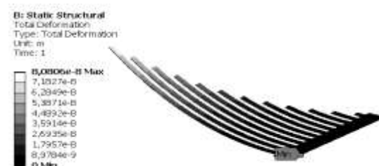
Рис. 5. Механическая деформация биматериальных консолей при \Delta T = 1^\circ \text{C}
