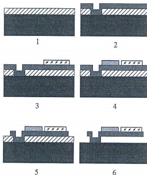
Рис.2. Основные технологические операции по изготовлению биматериальных неохлаждаемых ИК-приемников МОМС: 1 – осаждение жертвенного слоя \text{SiO}_2 ; 2 – травление окон в жертвенном слое для создания анкеров, осаждение слоя \text{Si}_3\text{N}_4 ; 3 – напыление слоя NiCr и его травление (формирование отражающего зеркала); 4 – напыление слоя Al и его травление (формирование биматериальной части консоли); 5 – травление слоя \text{Si}_3\text{N}_4 (формирование геометрии мембраны); 6 – удаление жертвенного слоя \text{SiO}_2
