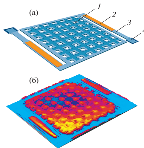
Рис. 1. Неохлаждаемый биматериальный чувствительный элемент и.к.-матрицы МЗ-50 размером 50 \times 50 мкм: а — конструкция чувствительного элемента (1 — приемная мембрана-зеркало, 2 — биматериальный участок микроконсоли, 3 — термоизоляционный участок микроконсоли, 4 — место крепления микроконсоли к подложке (якорь)); б — изображение чувствительного элемента, полученное на оптическом профилометре Wyko NT9300 (увеличение 101\times , режим вертикальной сканирующей интерферометрии высокого разрешения, сшивка).
